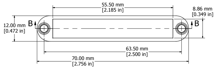
OPEN BEZEL
