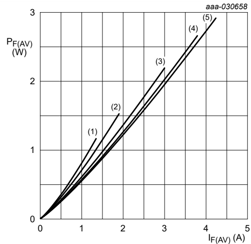
T_j = 175^\circ\text{C} (1) \delta = 0.1 (2) \delta = 0.2 (3) \delta = 0.5 (4) \delta = 0.8 (5) \delta = 1 ; DC
