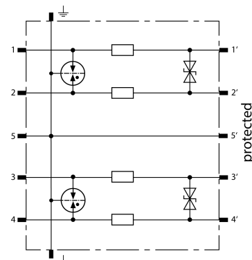
Prinzipschaltbild
