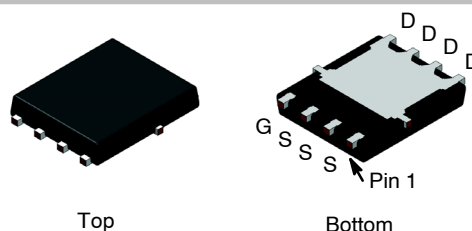
PQFN8 5x6 (Power 56) CASE 483AE
