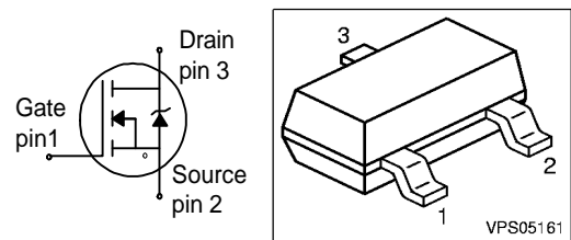
PG-SOT-23
