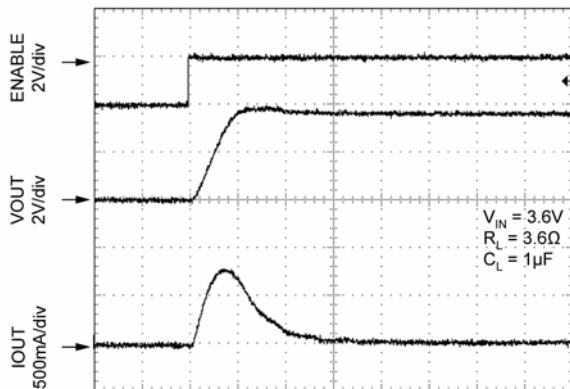
TIME 4µs/div
